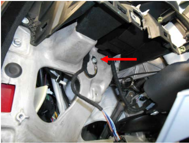
Выкрутить саморез.
